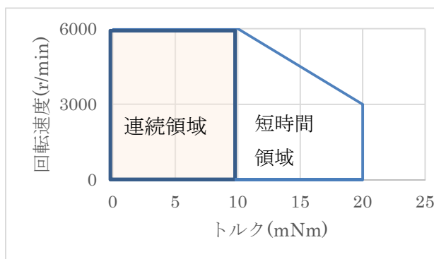
モータの運転領域 (SL22R, A1-SL22R 共通)
