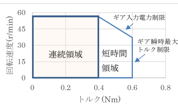
ギアモータ運転領域 (A1-SL22RG107P)
